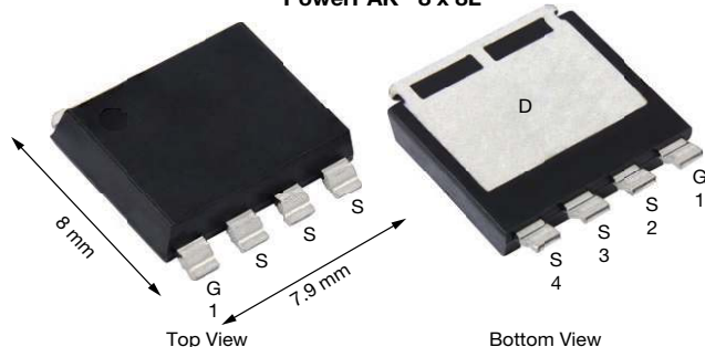
PowerPAK® 8 x 8L
