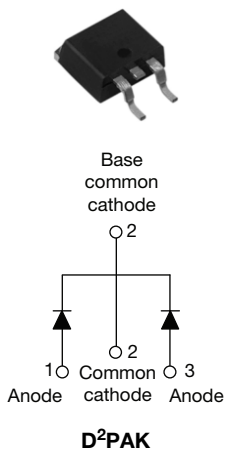
VS-16CTQ...GSPbF
