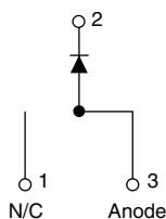
VS-15ETX06-1PbF
