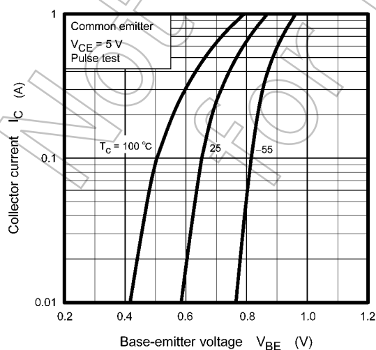
Fig. 7.5 I_C - V_{BE}
