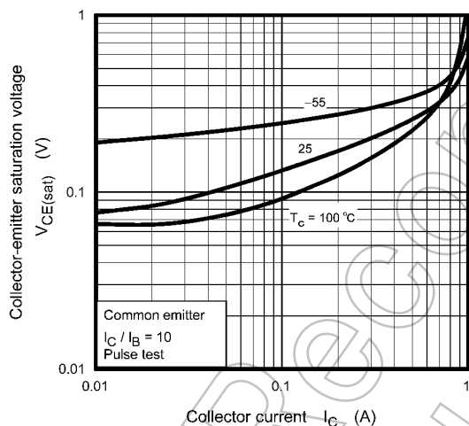
Fig. 7.3 V_{CE(sat)} - I_C
