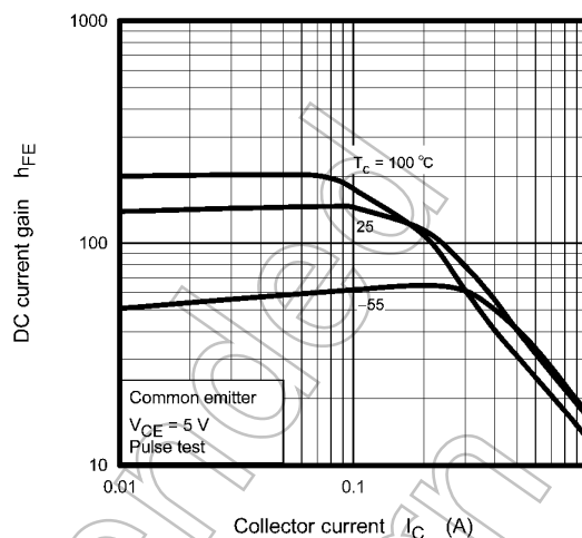
Fig. 7.2 h_{FE} - I_C
