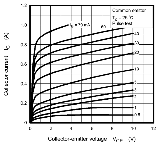
Fig. 7.1 I_C - V_{CE}
