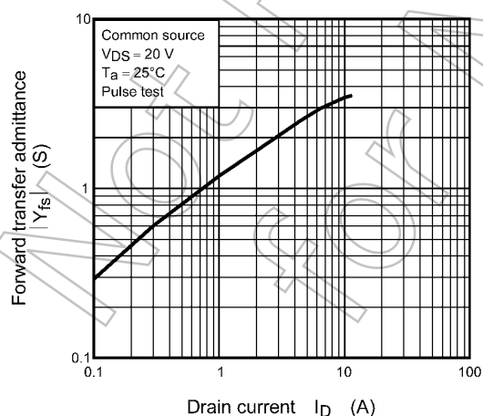
Fig. 8.5 |Y_{fs}| - I_D
