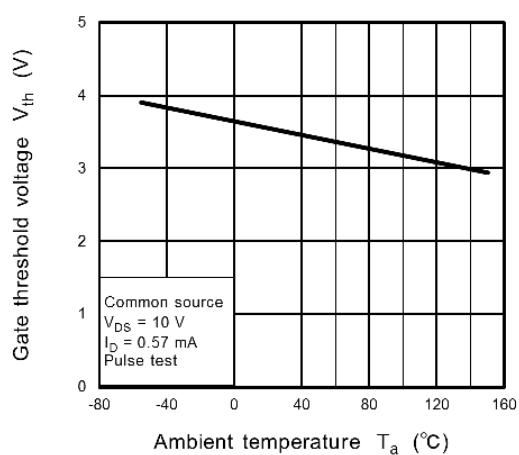
Fig. 8.11 V_{th} - T_a
