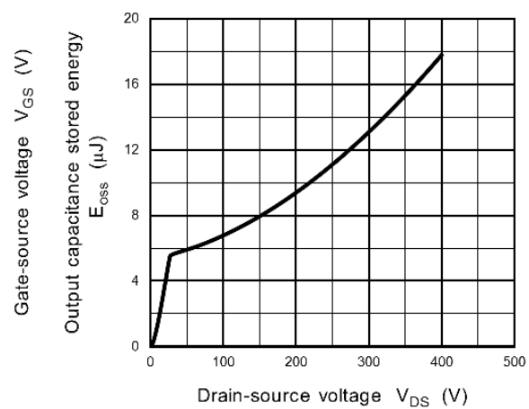
Fig. 8.12 E_{oss} - V_{DS}
