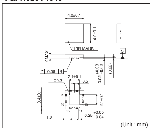
VQFN020V4040
