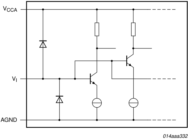
Fig 10. Analog inputs
