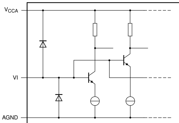
Fig 10. Analog inputs
