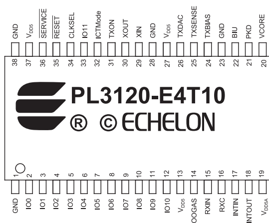
38 Pin TSSOP
