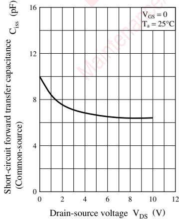
C_{iss} - V_{DS}
