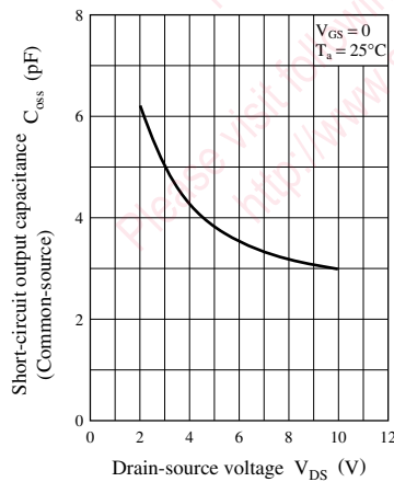
C_{oss} - V_{DS}
