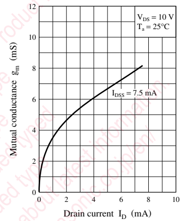
g_m - I_D
