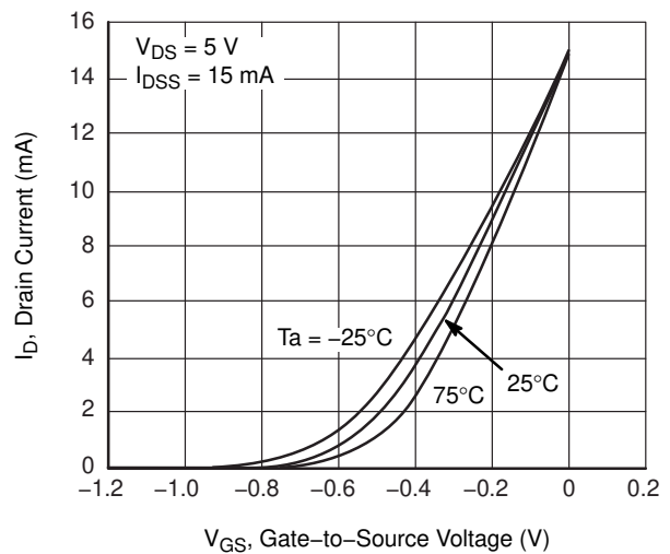
Figure 4. I_D - V_{GS}
