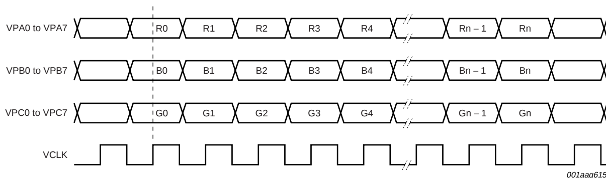
Fig 11. RGB 4 : 4 : 4 format data timing
