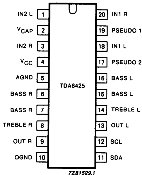
Fig.2 Pinning diagram.
