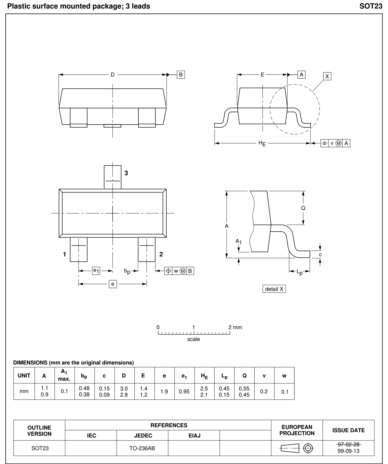
Fig 14. SOT23.
