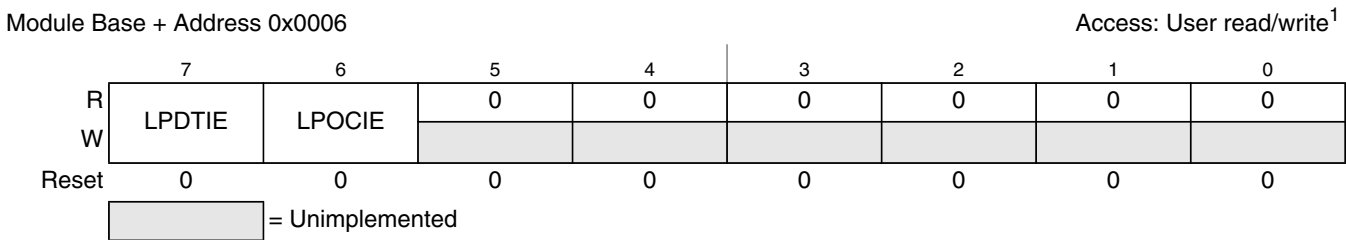
Figure 15-9. LIN Interrupt Enable Register (LPIE)
