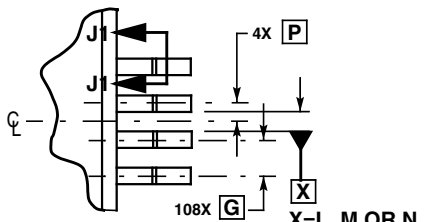
VIEW Y
