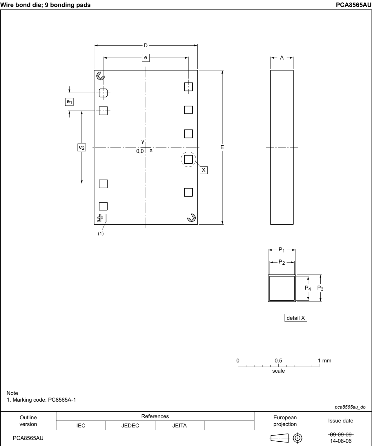
Fig 24. Bare die outline
