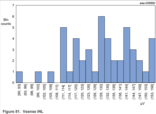
Figure 81. Vsense INL
