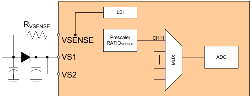
Figure 42. VSENSE Module
