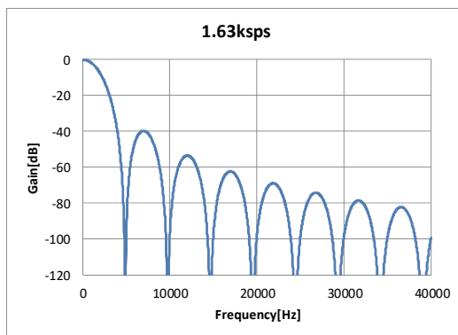
DR=1.63ksps
