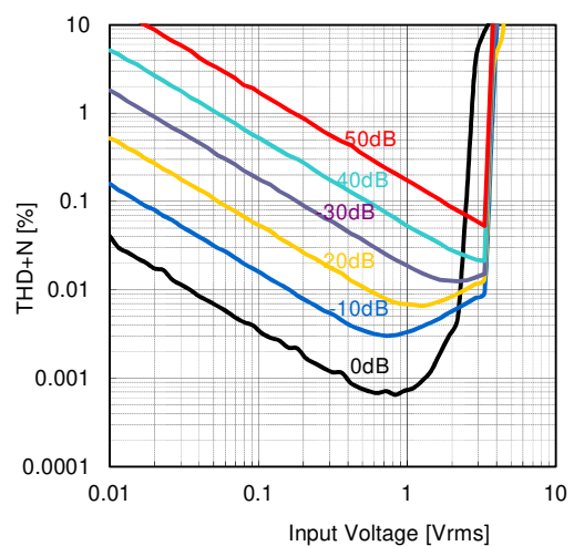
THD+N vs V_{in} -Volume V^+=9V , T_a=25^\circ C , f=1kHz , BW=400Hz-30kHz
