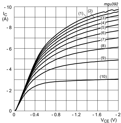
T_{amb} = 25^\circ\text{C} (1) I_B = -150\text{ mA} (2) I_B = -135\text{ mA} (3) I_B = -120\text{ mA} (4) I_B = -105\text{ mA} (5) I_B = -90\text{ mA} (6) I_B = -75\text{ mA} (7) I_B = -60\text{ mA} (8) I_B = -45\text{ mA} (9) I_B = -30\text{ mA} (10) I_B = -15\text{ mA}
