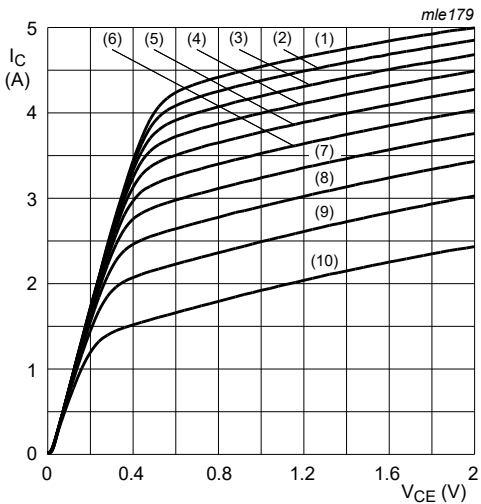
T_{amb} = 25^\circ\text{C} (1) I_B = 120\ \text{mA} (2) I_B = 108\ \text{mA} (3) I_B = 96\ \text{mA} (4) I_B = 84\ \text{mA} (5) I_B = 72\ \text{mA} (6) I_B = 60\ \text{mA} (7) I_B = 48\ \text{mA} (8) I_B = 36\ \text{mA} (9) I_B = 24\ \text{mA} (10) I_B = 12\ \text{mA}
