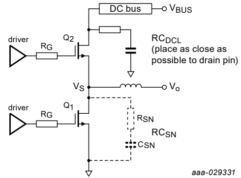
Fig. 16. DC-link snubber circuit
