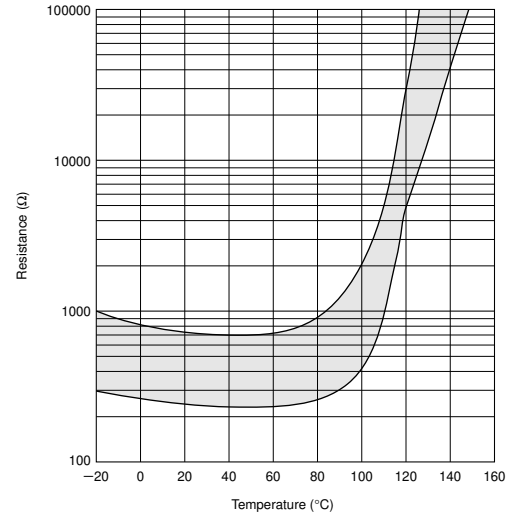
PRF15BB471QB1RC
