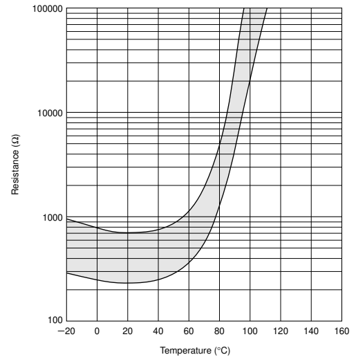
PRF18/21BE471Q Type
