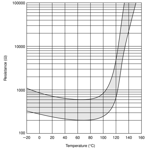
PRF18/21AS471Q Type
