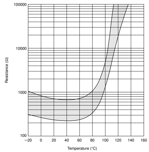
PRF18/21BA471Q Type
