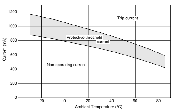
PTGL09AS1R2K2B51B0
