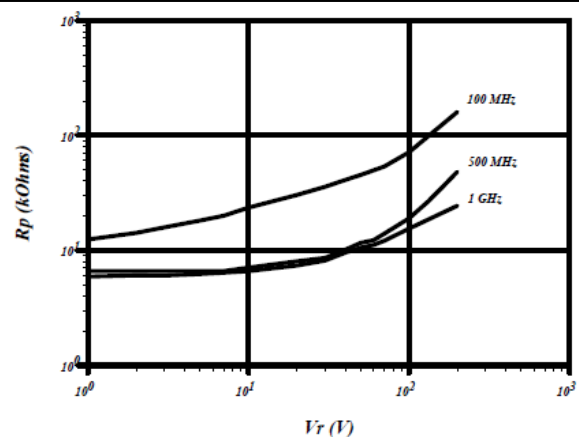
R_P VS V_R (UM4300)
