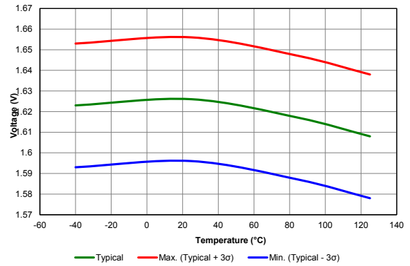
Figure 40-64. POR RELEASE VOLTAGE, (VREGPM = 'b0x)
