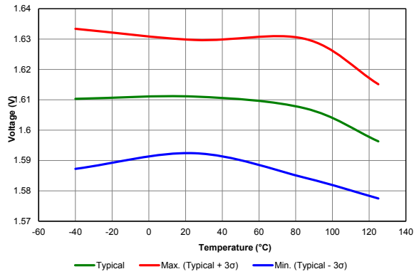
Figure 40-65. POR REARM VOLTAGE, (VREGPM = 'b1x)
