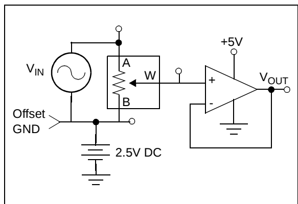
2.1 Test Circuits
