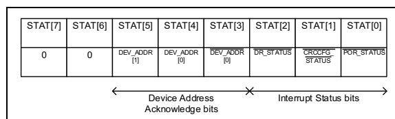
FIGURE 6-1: STATUS Byte.
