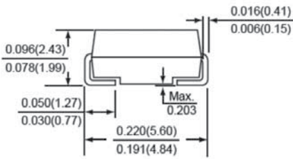
SMA/DO-214AC
