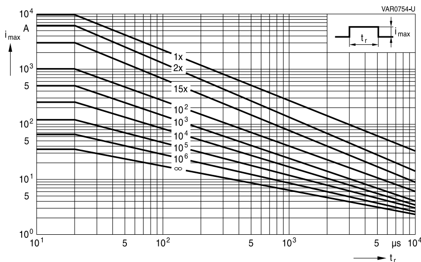
SIOV-SNF20K350 ... K625E2S5K1
