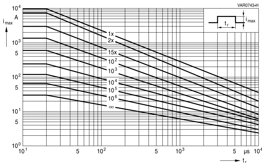
SIOV-SNF20K130 ... K320E2S5K1
