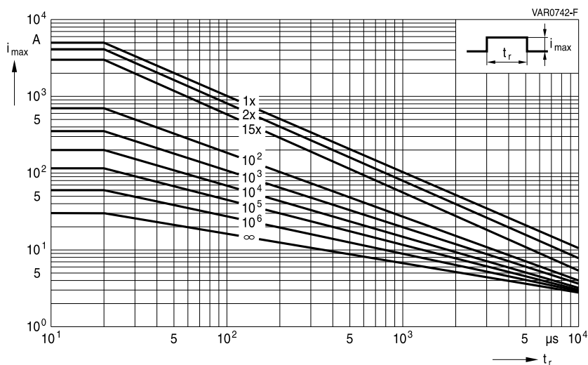
SIOV-SNF14K350 ... K625E2S5K1
