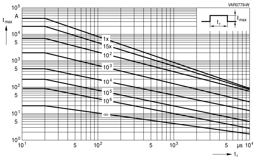
SIOV-LS40K130QP(K2) ... K150QP(K2)
