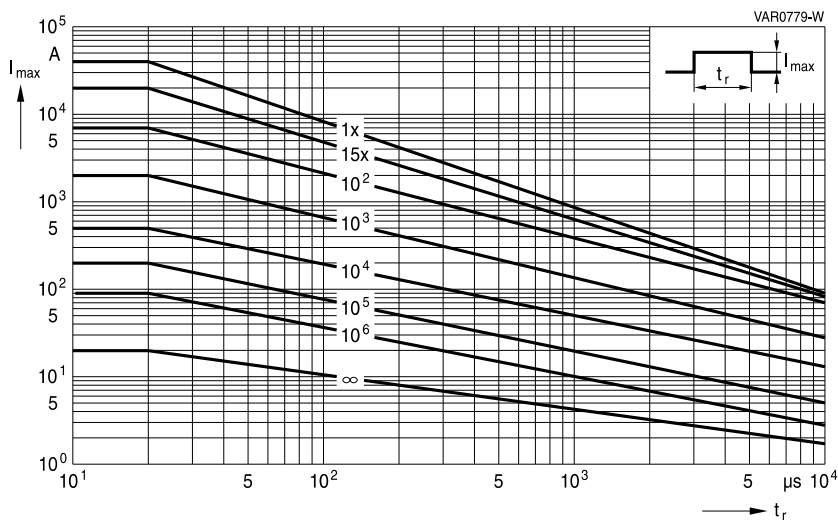
SIOV-LS40K130QP(K2) ... K150QP(K2)
