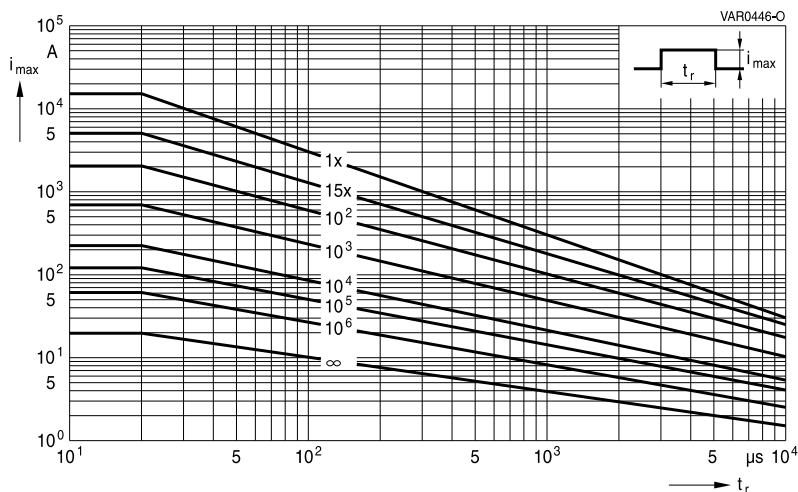
SIOV-Q20K130 ... K320
