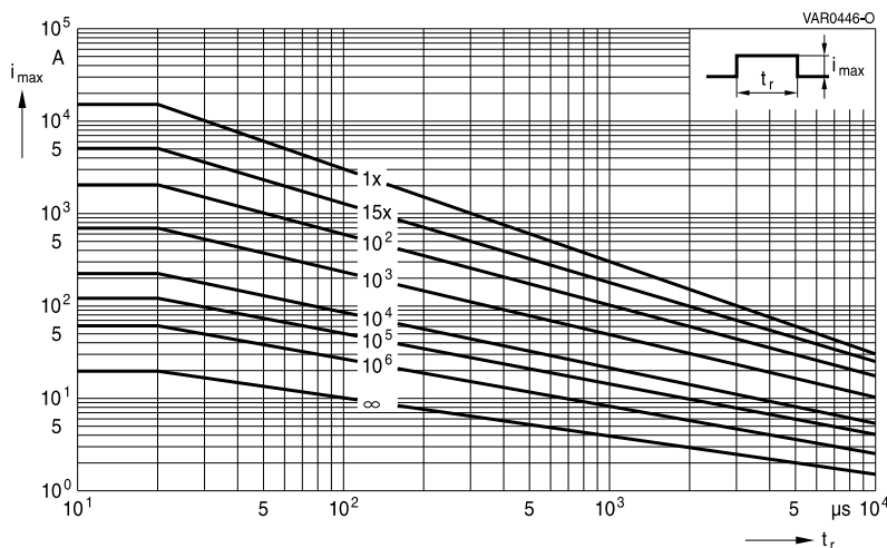
SIOV-Q20K130 ... K320
