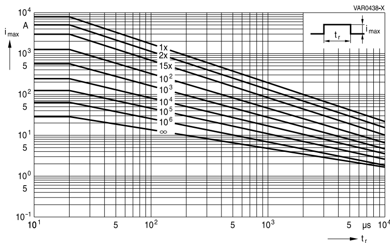
SIOV-Q14K130 ... K320
