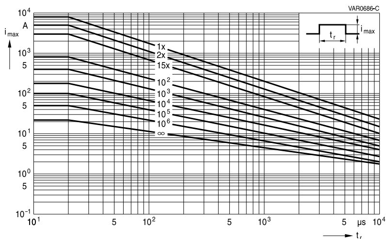
SIOV-Q14K350 ... K460
