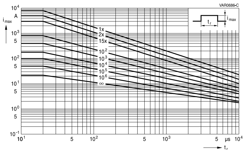
SIOV-Q14K350 ... K460
