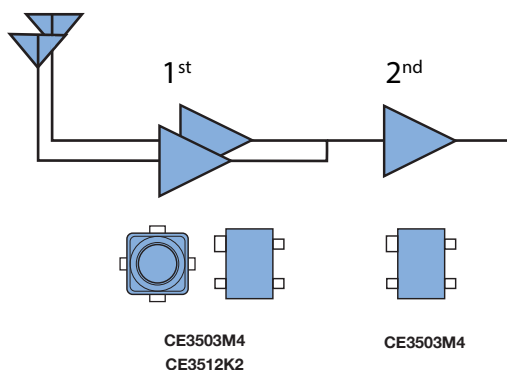
12GHz LNB
