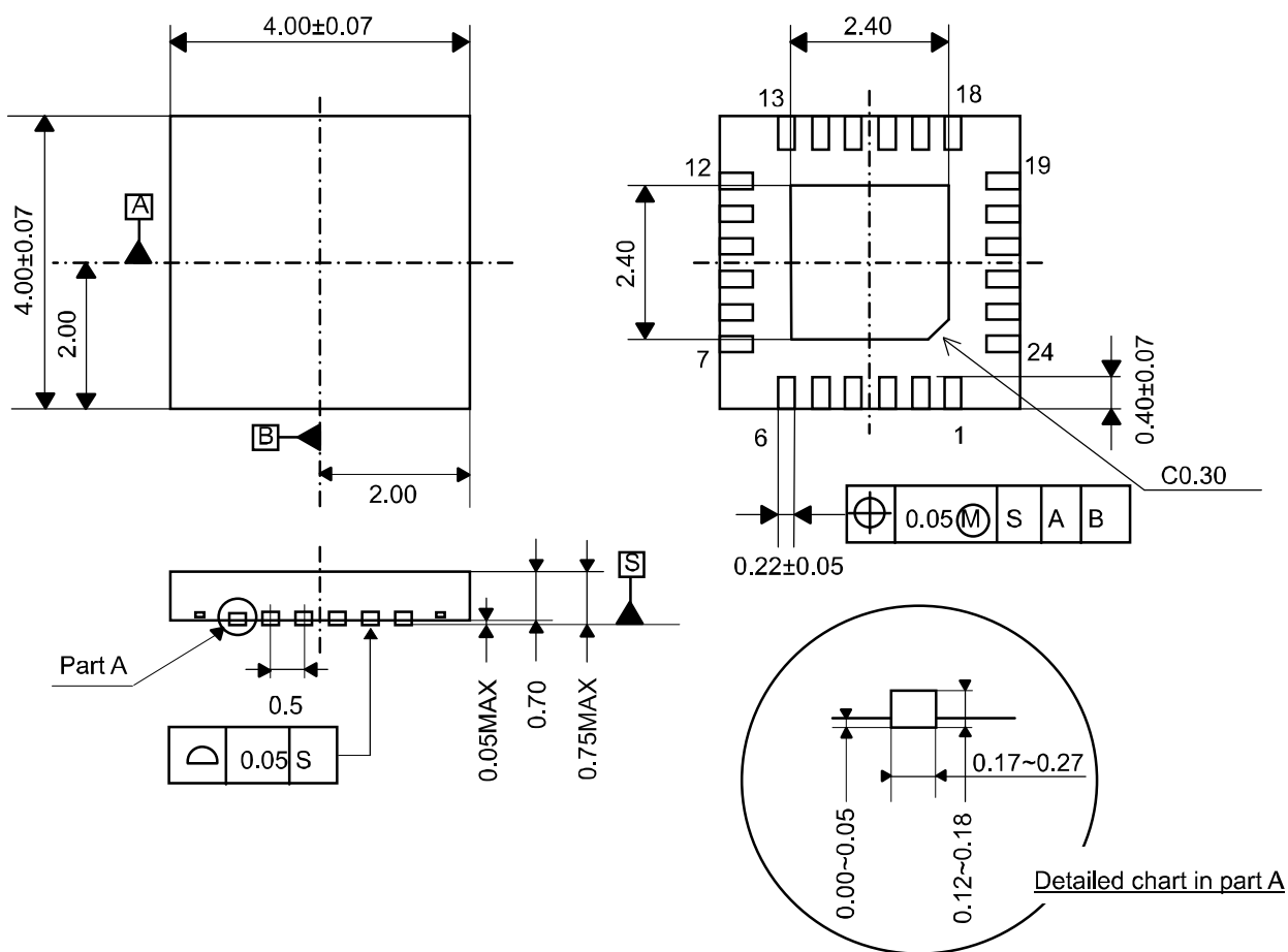
Fig. 15 Outer Dimensions
