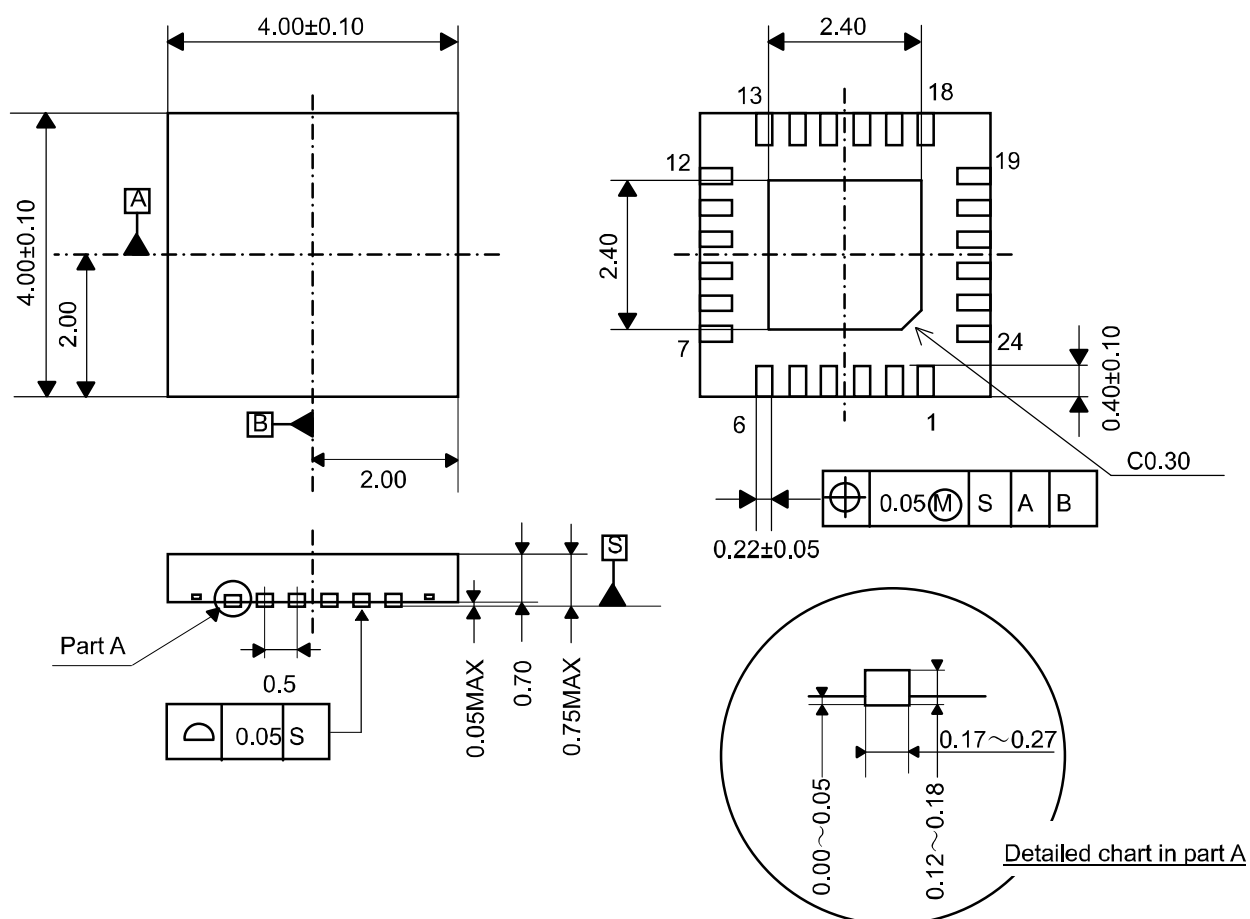
Fig. 16 Outer Dimensions
