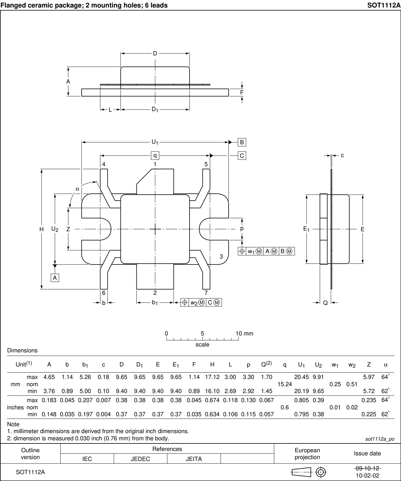
Fig 14. Package outline SOT1112A
